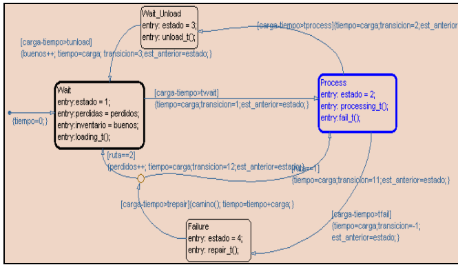
Fig. 7. Implementación en STATEFLOW de la máquina de carga descarga.
