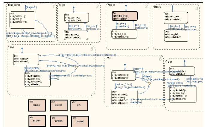
Fig. 10. Implementación del Servidor de Archivos (Stateflow)
