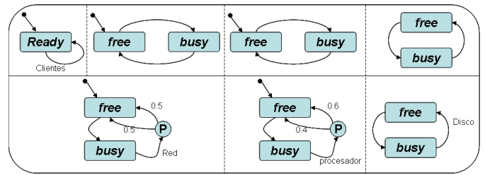
Fig. 9. Diagrama statechart del servidor
