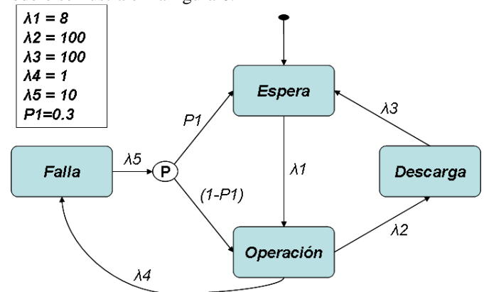
Fig. 6. Statechart de la máquina de carga/descarga..
