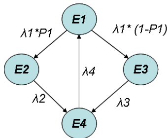
Fig. 5. Cadena de Markov correspondiente al diagrama de la figura 4.
