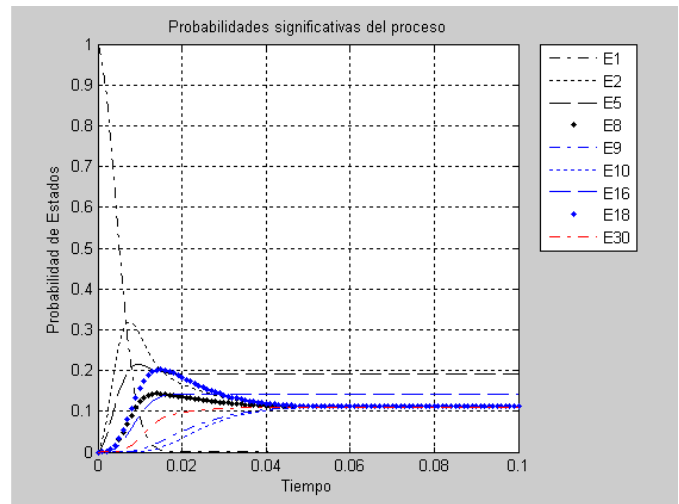
Fig. 14. Utilización del procesador
